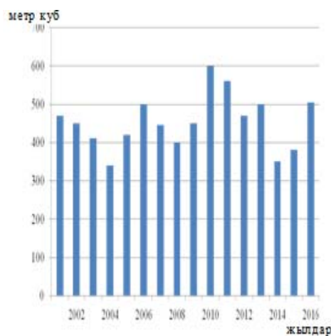
1-сурет – Қапшағай суқоймасының су деңгейі режимінің динамикасы мен Іле өзенінің жылдық орташа су шығынының динамикасы: а – Қапшағай суқоймасы; б – Іле өзені
